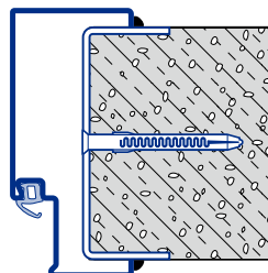
Umfassungszarge B73 Schweißmontage D Typ 2
