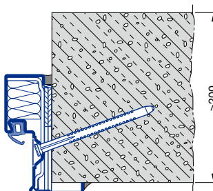
DryFix Zarge Diagonalfestigung B Typ 1
