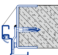
Eckzarge Schweißmontage A Typ 2 / A Typ 3
