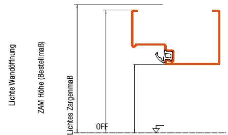
4-seitig umlaufende Zarge (Tür) ZAM Breite ZAM Höhe
