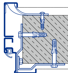
Eckzarge mit Ergänzungszarge Dübelmontage C Typ 3
