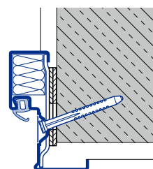
DryFix Zarge Diagonalfestigung B Typ 1
