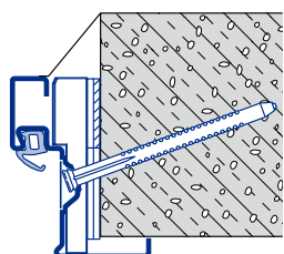
Eckzarge Diagonalfestigung A Typ 1
