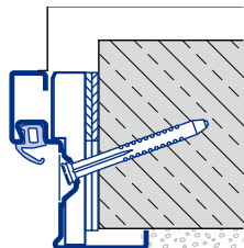
Eckzarge Diagonalfestigung A Typ 1
