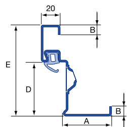
Eckzarge Diagonalbefestigung
